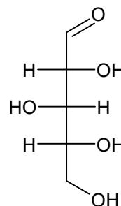
D-xylóza
