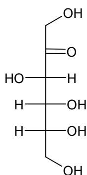
D-fruktóza
