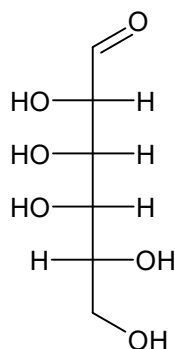
D-talóza
