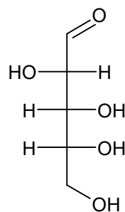
D-arabínóza
