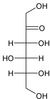
D-sorbóza
