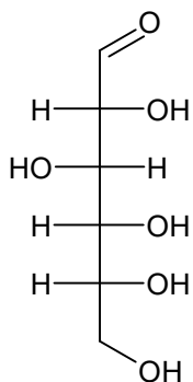
D-glukóza
