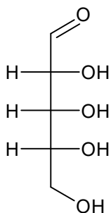
D-riboza
