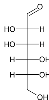
D-manóza
