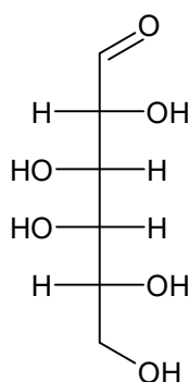
D-galaktóza
