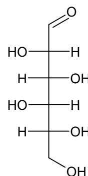
D-idóza
