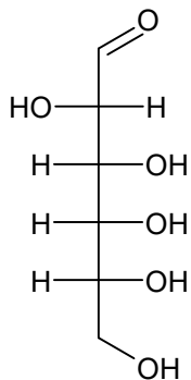
D-altróza
